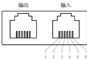
RJ12 接口
