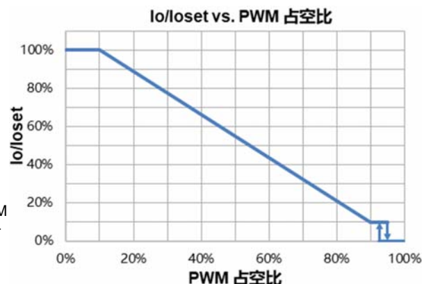
示意图 4: 负逻辑
