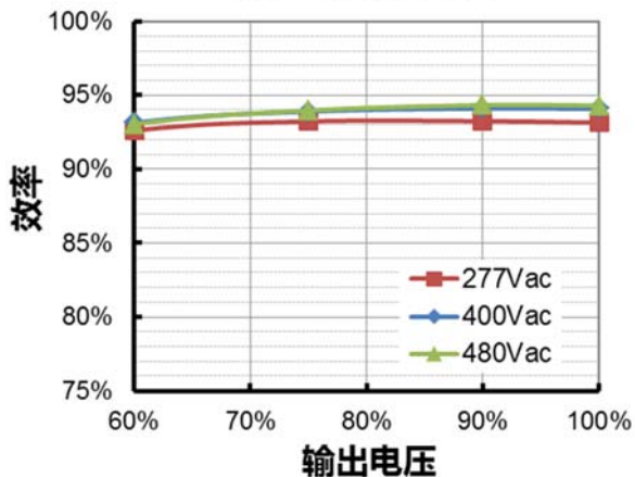
ESM-320S250Lx( I_o=1750mA ) 效率 vs. 输出电压
