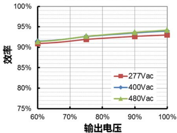
ESM-320S250Lx( I_o=2500mA ) 效率 vs. 输出电压
