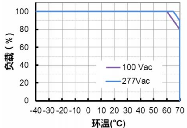
降额曲线
