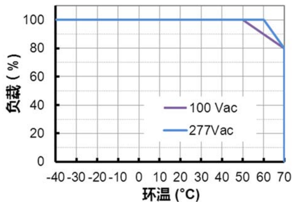
降额曲线
