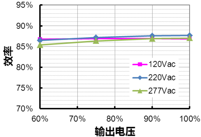
EUC-040S070DTM0004( I_o=500mA ) 效率 vs. 输出电压
